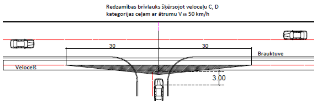
Redzamības brīvlauks E kategorijas ceļam ar ātrumu V_{as} 20 km/h
