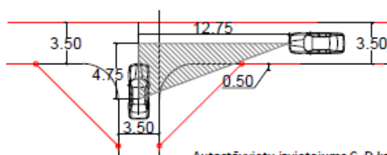
Autostāvvietu izvietojums C, D kategorijas ielai ar ātrumu V_{as} \leq 50 km/h
