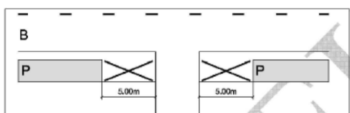
Autostāvvietu izvietojums C, D kategorijas ielai ar ātrumu V_{as} \leq 50 km/h
