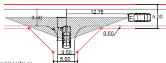
Redzamības brīvlauks D, E kategorijas ceļam ar ātrumu V_{as} 30 km/h
