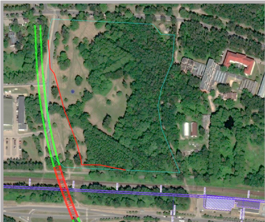
5. attēls. Dzelzceļa infrastruktūras Rail Baltica projekta risinājumi dzelzceļa šķersojumam pie Anniņmuižas bulvāra. Tūneļa trasējuma uzmetums un aptuvenais šķērsojums. 2023. gada maijs.
