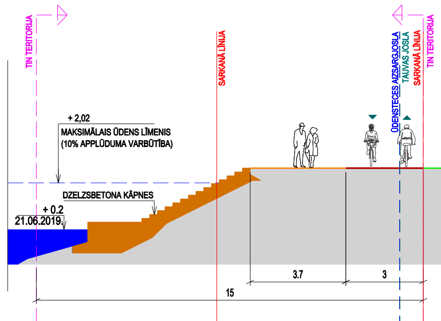
TERITORIJAS GRIEZUMS GRIEZUMS A - A
